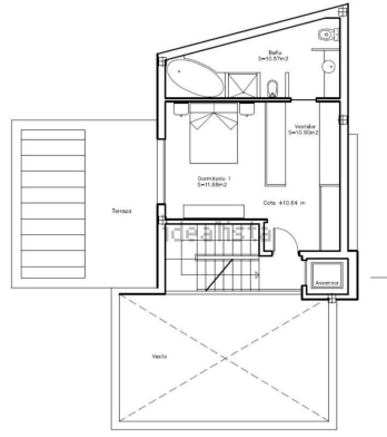
PLANTA ALTA 50,82 m 2
